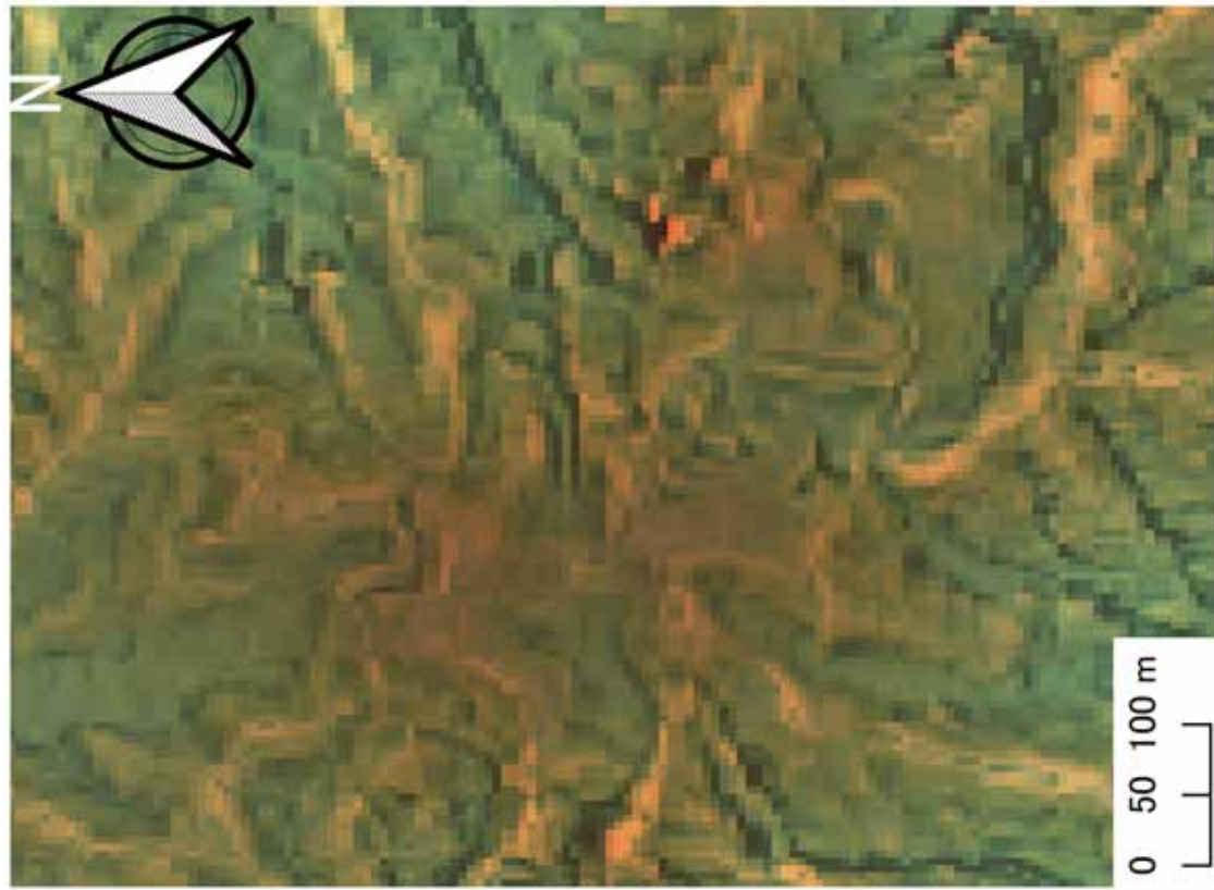
図1 城山城跡の5 mメッシュDEMから作成した立体図 (S=1/7000、国土地理院数値標高モデルFG-GML- 5234-24-DEM5Aから作成)
