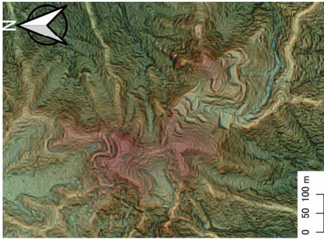
図2 城山城跡の1 mメッシュDEMから作成した立体図 (S=1/7000、兵庫県1 mメッシュDEM_alt_050E0 43および同044から作成)
